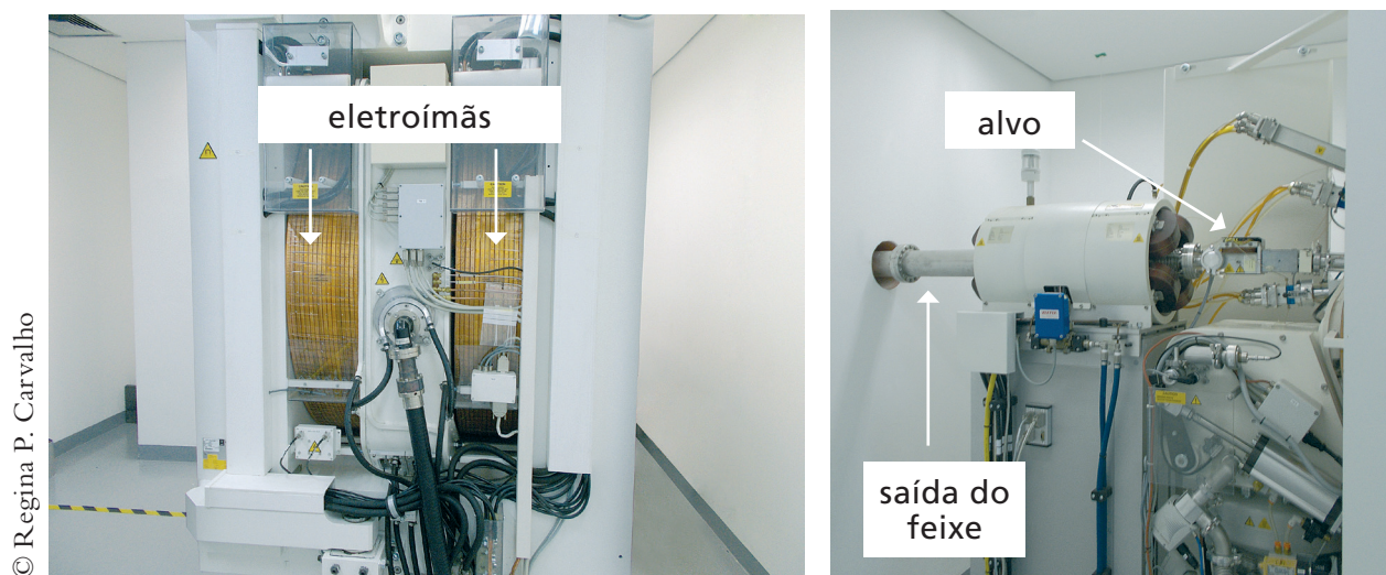
Figura II-3 – Ciclotron (CDTN-CNEN)
